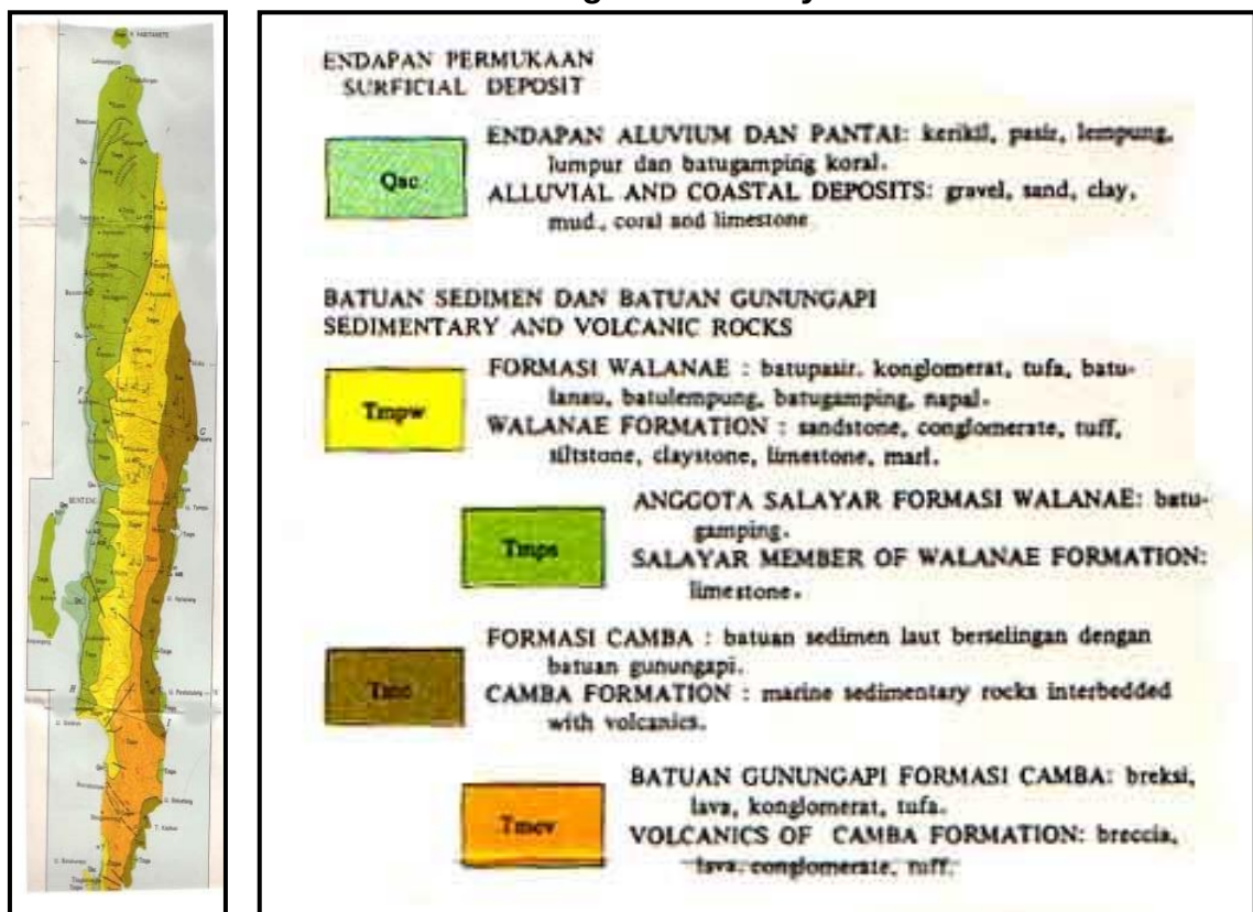
Gambar 2.2. Peta Geologi Pulau Selayar
